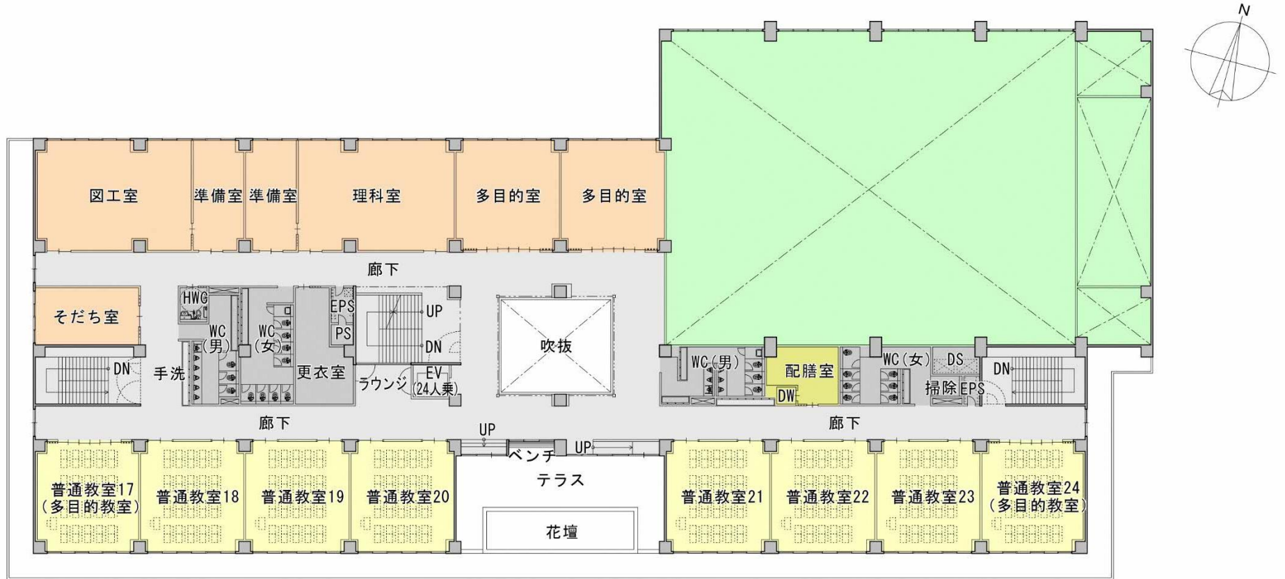
4階平面図 S:1/400
