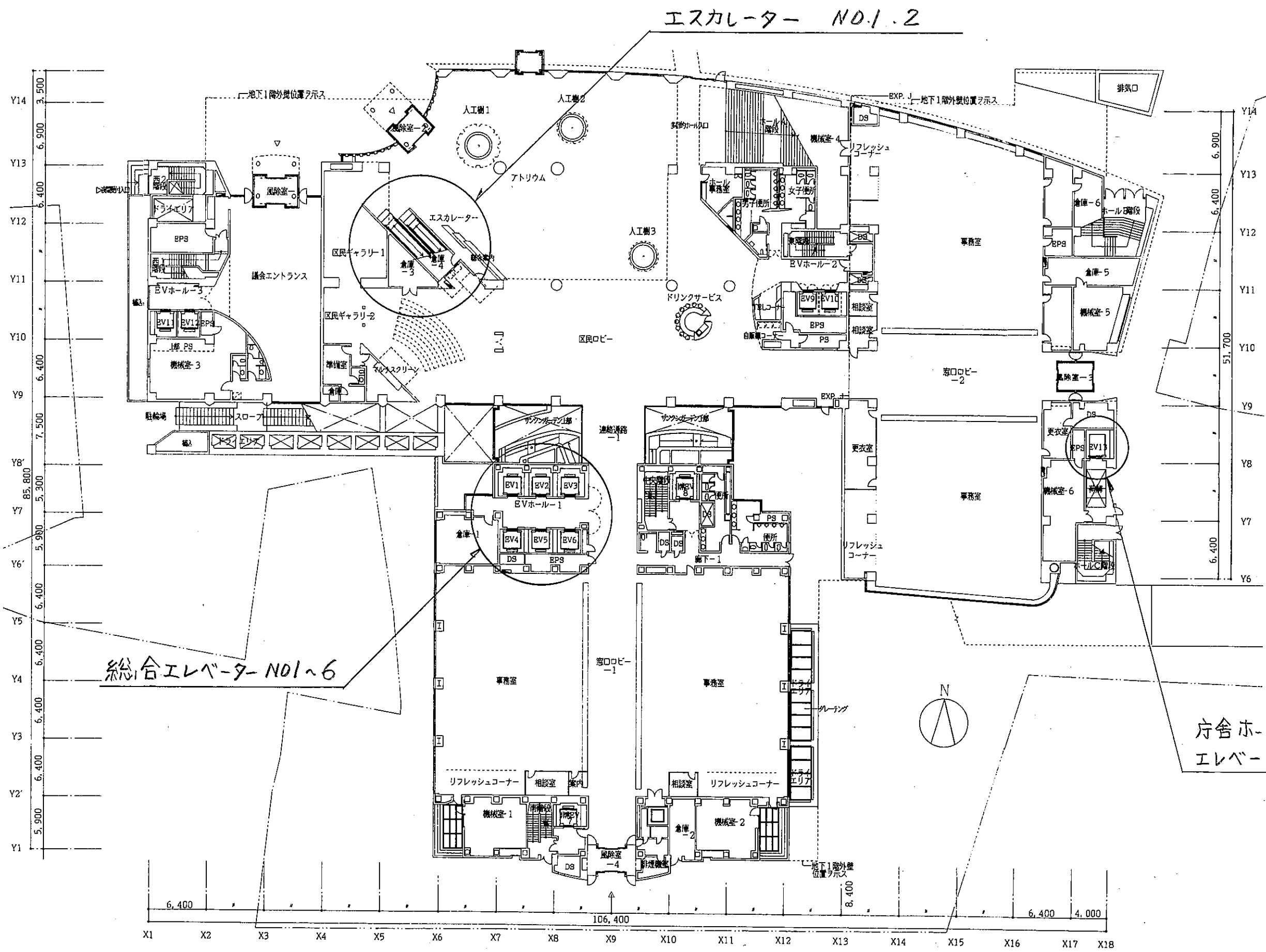
1階 平面図
