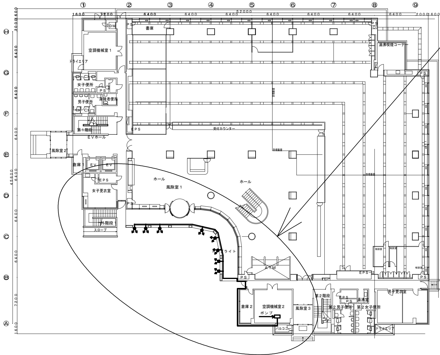
北館 1 階平面図
